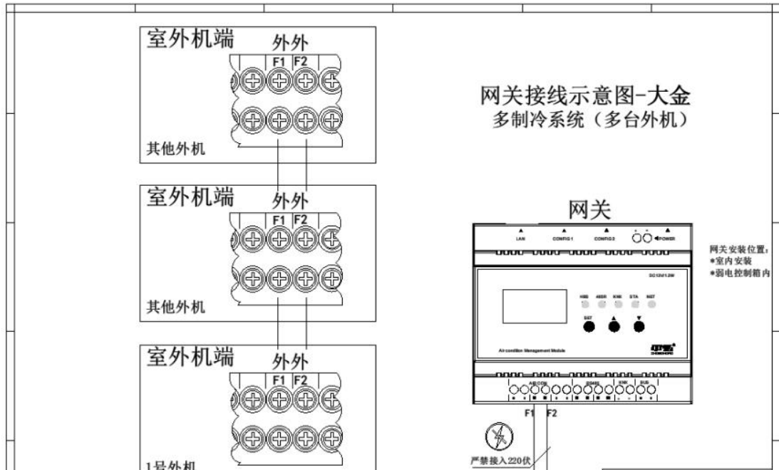
图 4 大金空调接线位置
