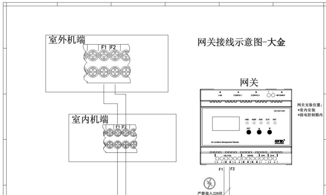
图 3 大金空调接线位置
