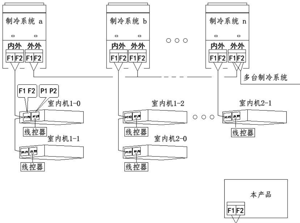
图 2 大金空调本产品系统接线方式
